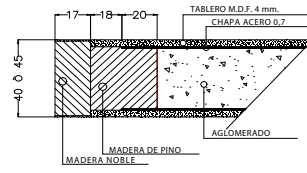
SECCIÓN BLINDADA C / O
