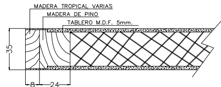
HUECA C / O. T / 5 mm.
