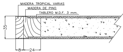
MACIZA C / O.
