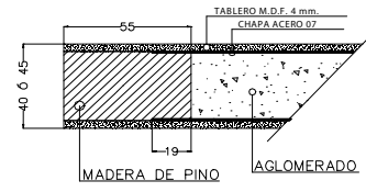
SECCIÓN BLINDADA C / PINO
