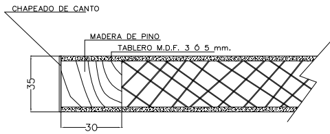
HUECA C / CHAPEADO
