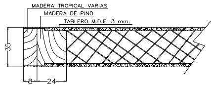
HUECA C / O
