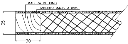
HUECA C / PINO
